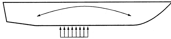
그림 3.2.9 중앙부 파정 착수
