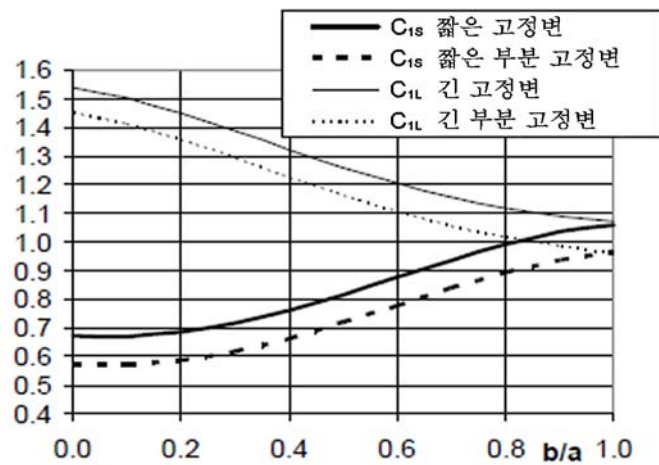
그림 3.5.5 계수 C_1
