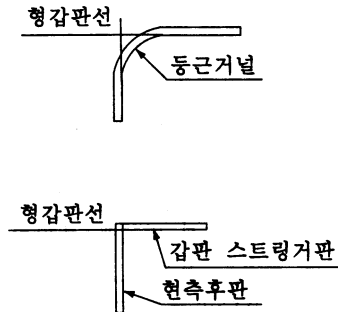
그림 3.3.3 형기준선
