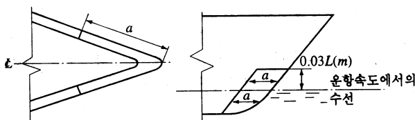
그림 3.5.1 충돌보호
