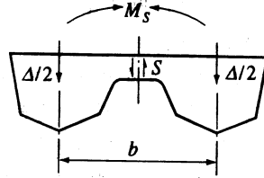
그림 3.2.12 횡방향 수직 굽힘모멘트 및 전단력
