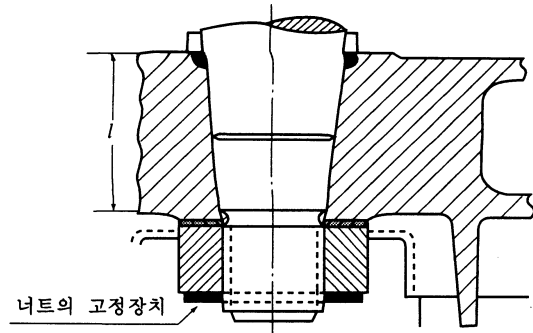
그림 4.1.4 유압장치를 가진 콘 커플링
